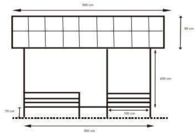
Tampak Depan
